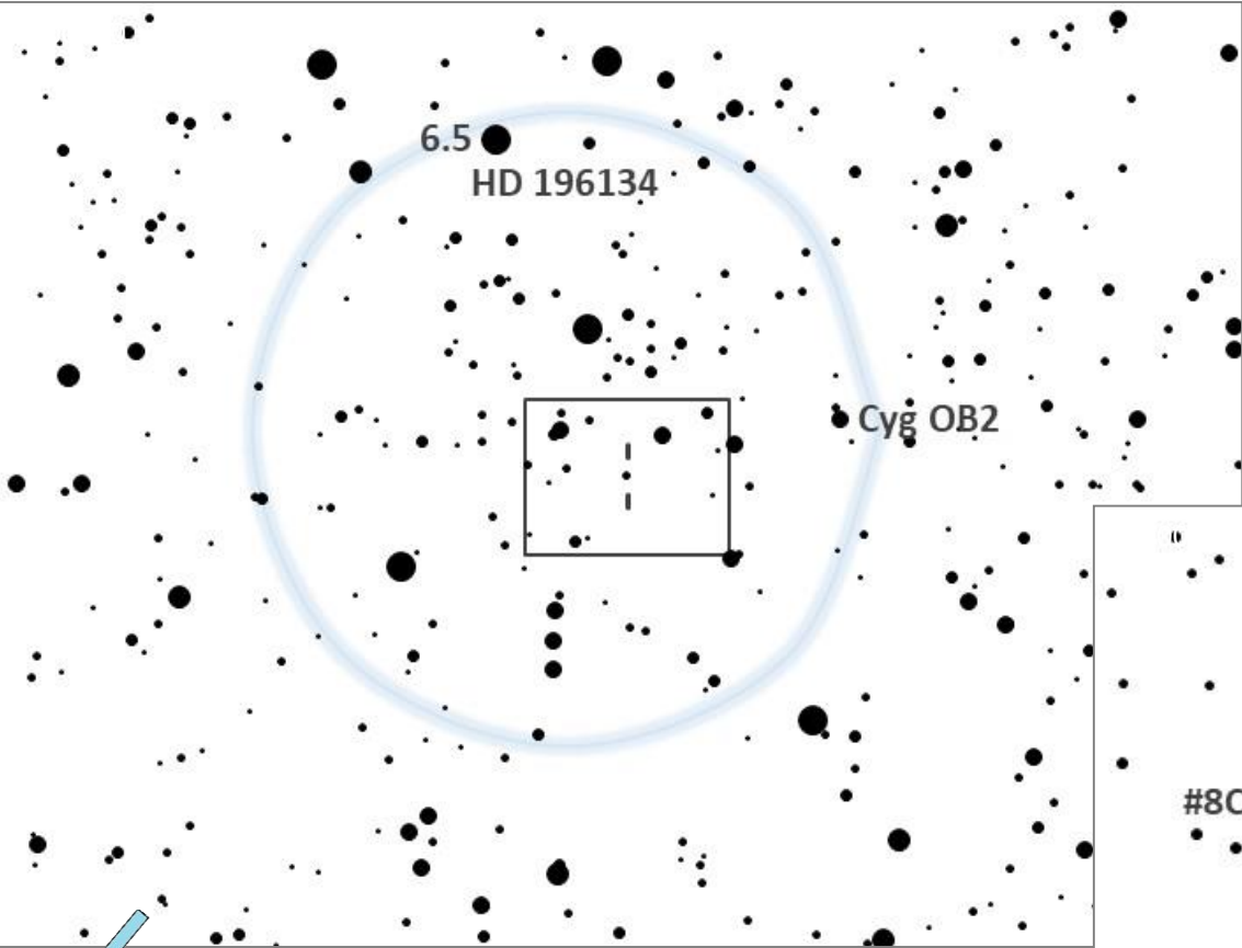
HIPPARCOS + Tycho2 , magnitude < 12.5
