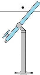
HIPPARCOS + Tycho2 , magnitude < 12.5
